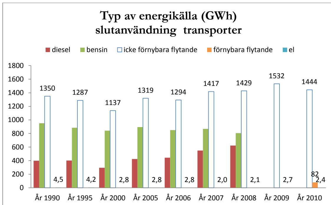
Figur 10. Slutanvändning för sektor transporter uppdelat på icke förnybara och förnybara energikällor och för åren 1990-2008 specificerat i diesel och bensin.
