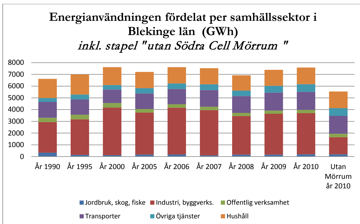
Figur 7. Slutlig energianvändning i Blekinge utan Södra Cell Mörrum.
